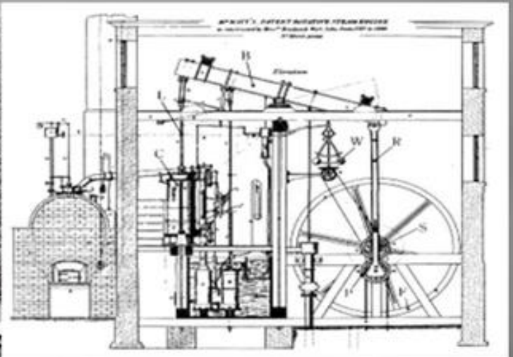
<증기기관 설계도>
